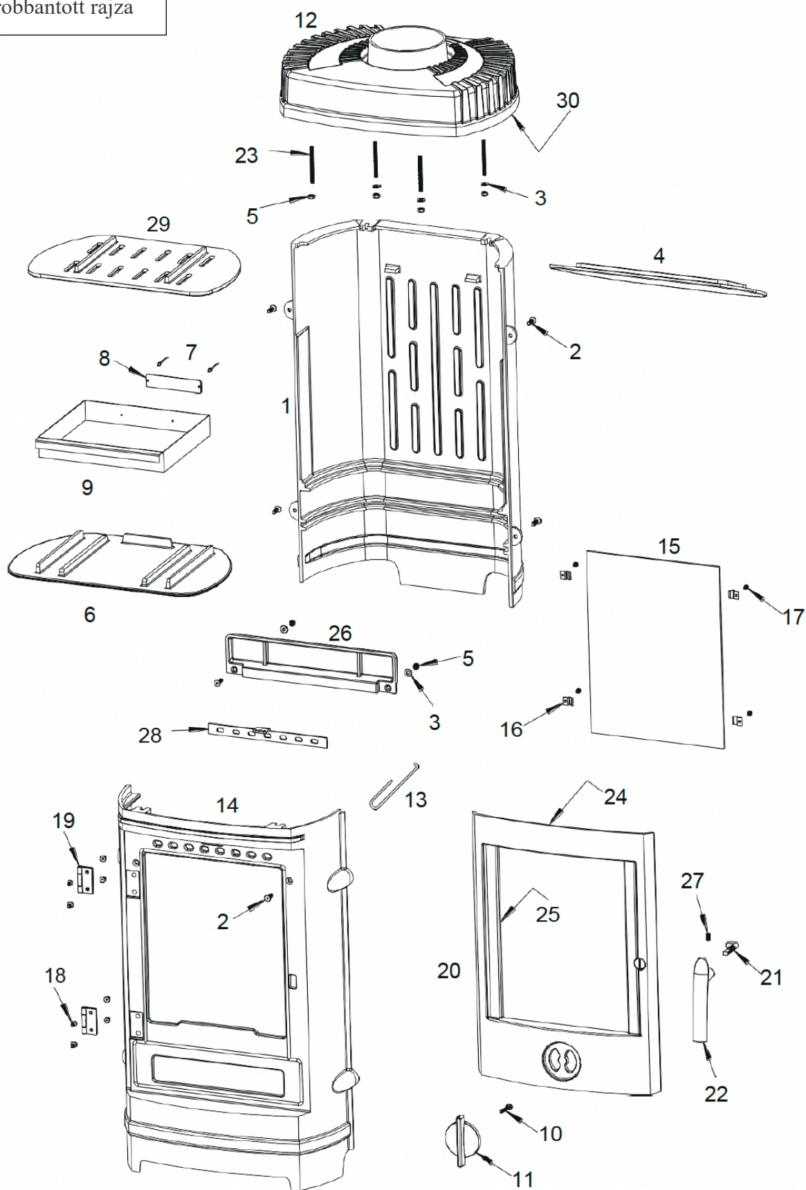
A készülék robbantott rajza
